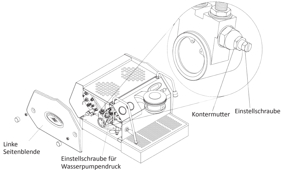
Abbildung 7 – Einstellen des Wasserpumpendrucks
