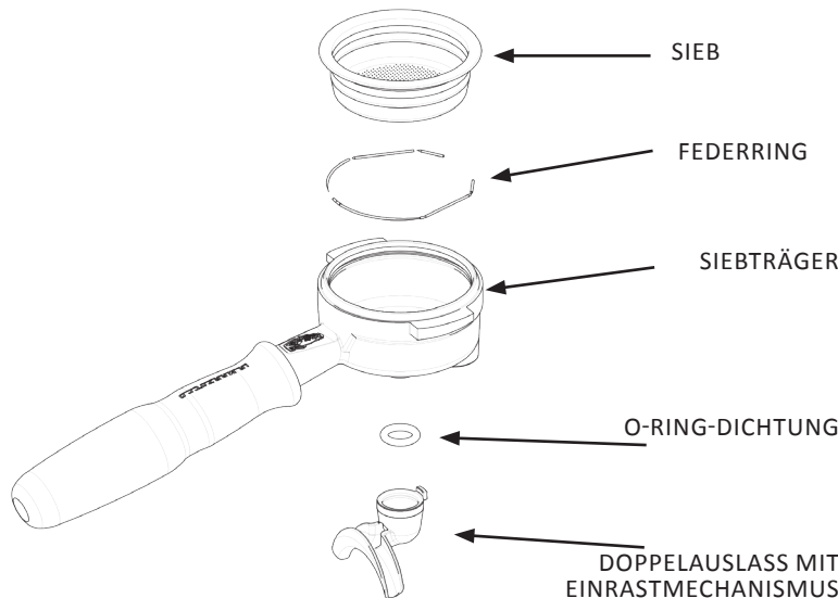
Abbildung 8 – Siebträger
